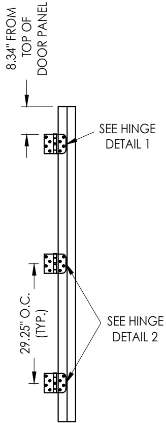
HINGE JAMB
